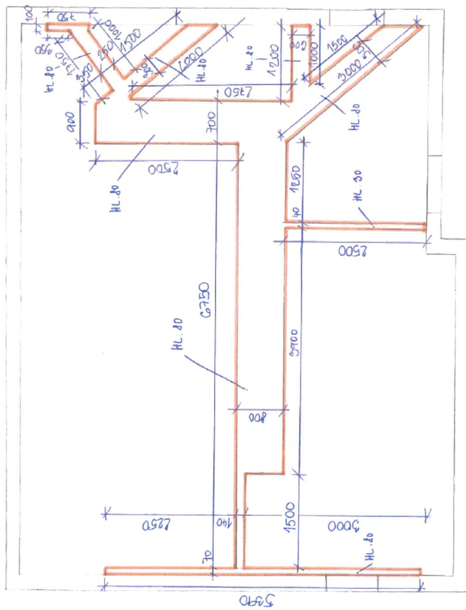
ZLG.1 - Drážky v podlaže – učebna fyziky
