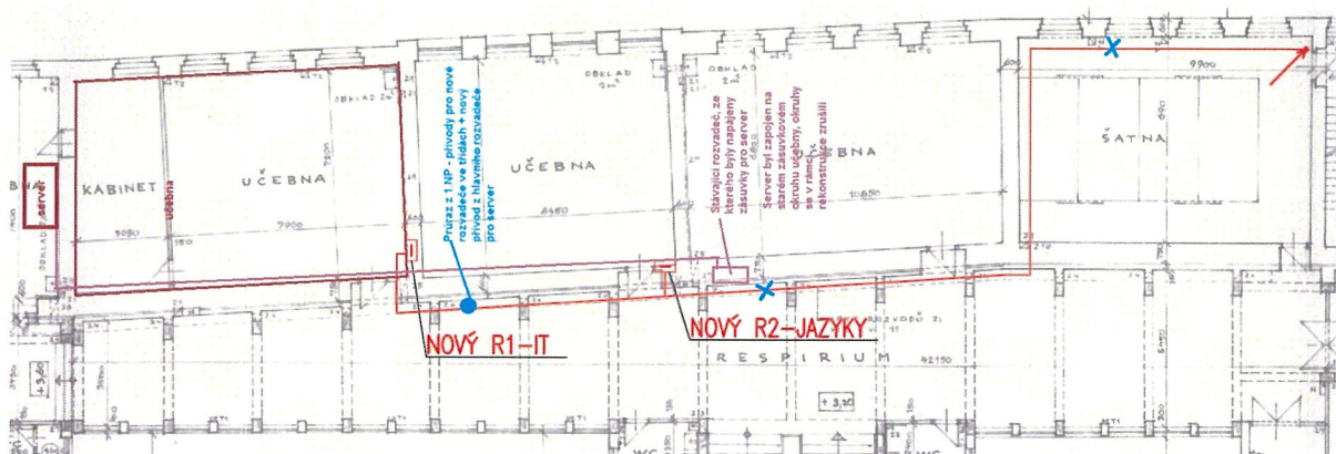
ZL 5.8 Výměna zárubní - jazyková učebna
